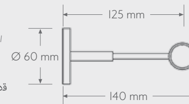
OKA 01 rustik ayağı bracket резная ножка قدم ريفي عادي
