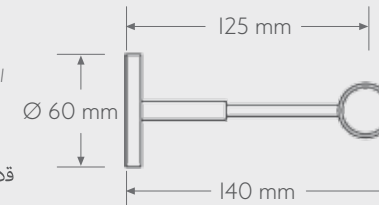
AKA 02 yan duvar aprt. side wall bracket appar. Боковая стенка جاذب جدار القدم
